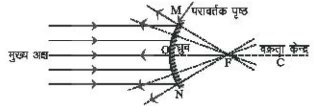
चित्र 9.8 (b) उत्तल दर्पण
