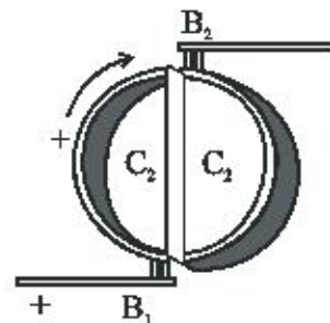
चित्र 10.14 दिष्टधारा जनित्र
