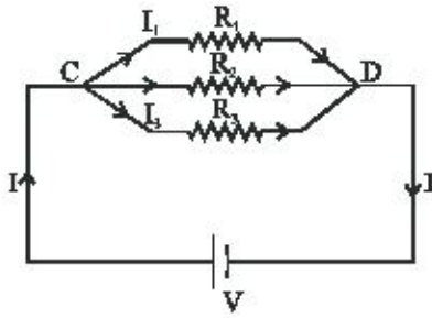
चित्र 10.8 प्रतिरोधों का समान्तर क्रम संयोजन ओम के नियम से
