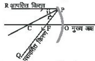
चित्र 9.8 अवतल दर्पण से परावर्तन
