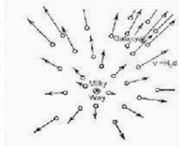
चित्र 18.3 बिगबैंग अवधारणा को प्रदर्शित करता रेखाचित्र
